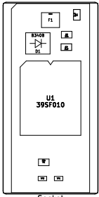
Socket
